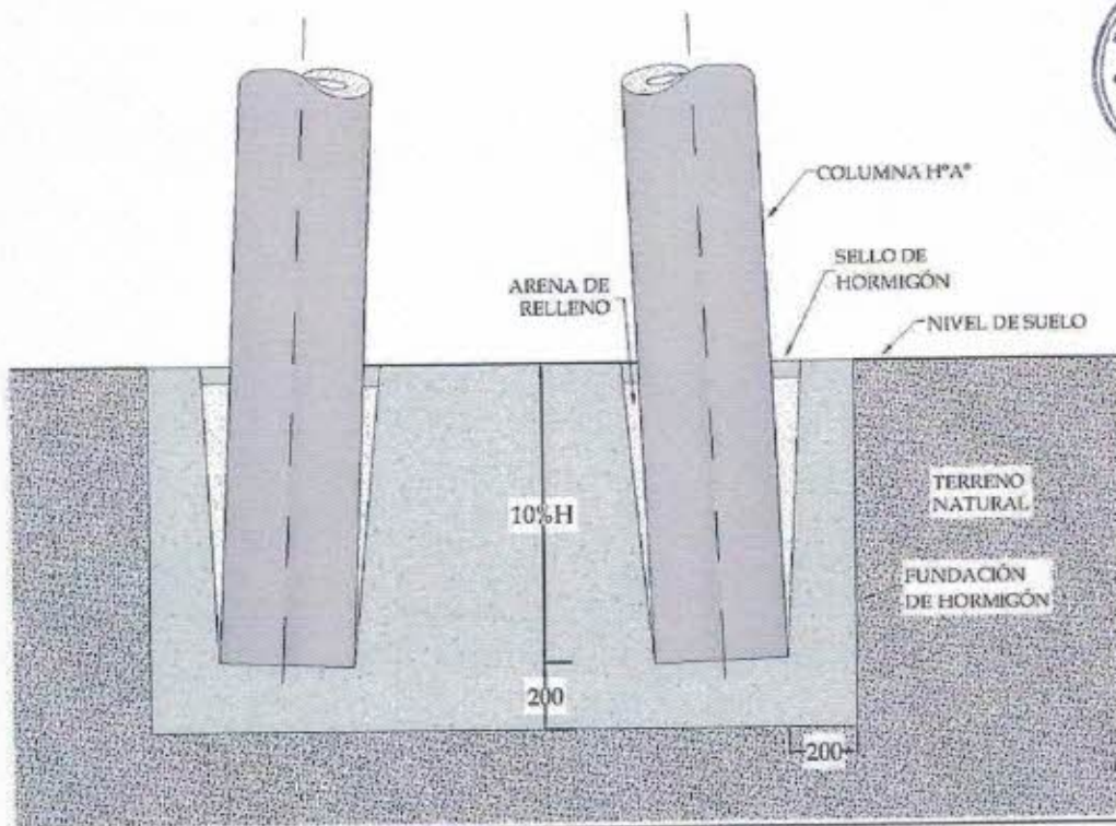
Fundación de Hormigón en Estructura Doble
