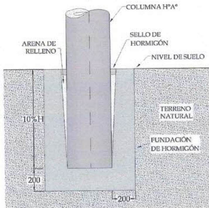
Fundación de Hormigón en Columna simple
